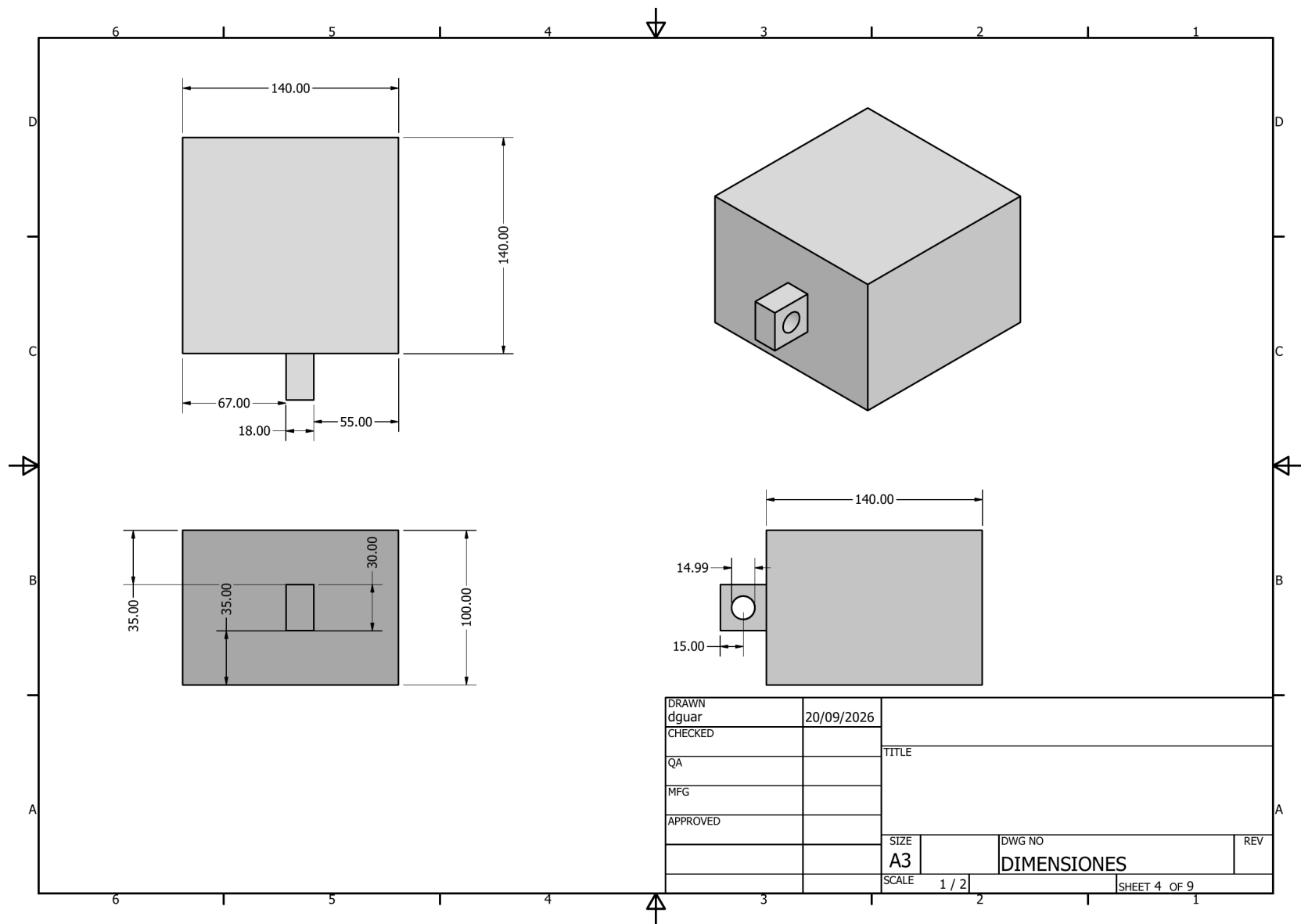
Figura 21. Hoja 4: Bloque (píson) (escala 1:2).
