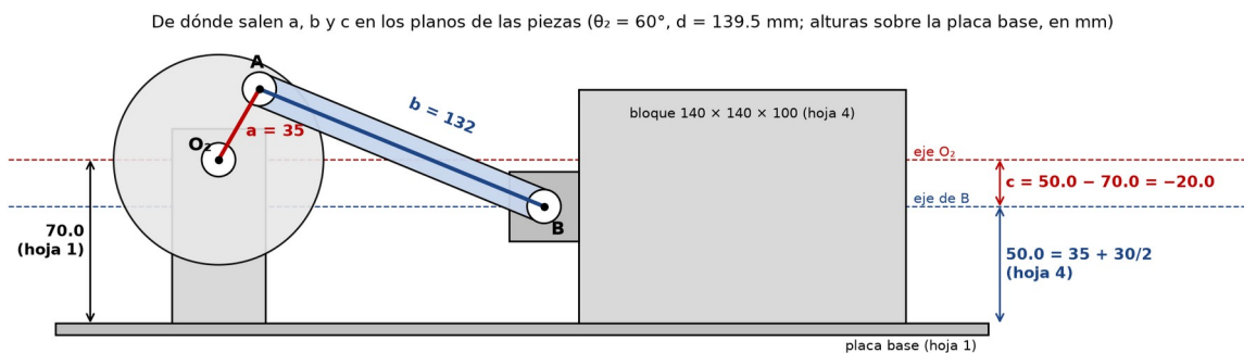
Figura 5. Cómo salen a, b y c de los planos: alturas del eje O 2 (soporte, hoja 1) y del pasador B (oreja del bloque, hoja 4) sobre la placa base. Dibujo a escala con \theta_2 = 60^\circ .
