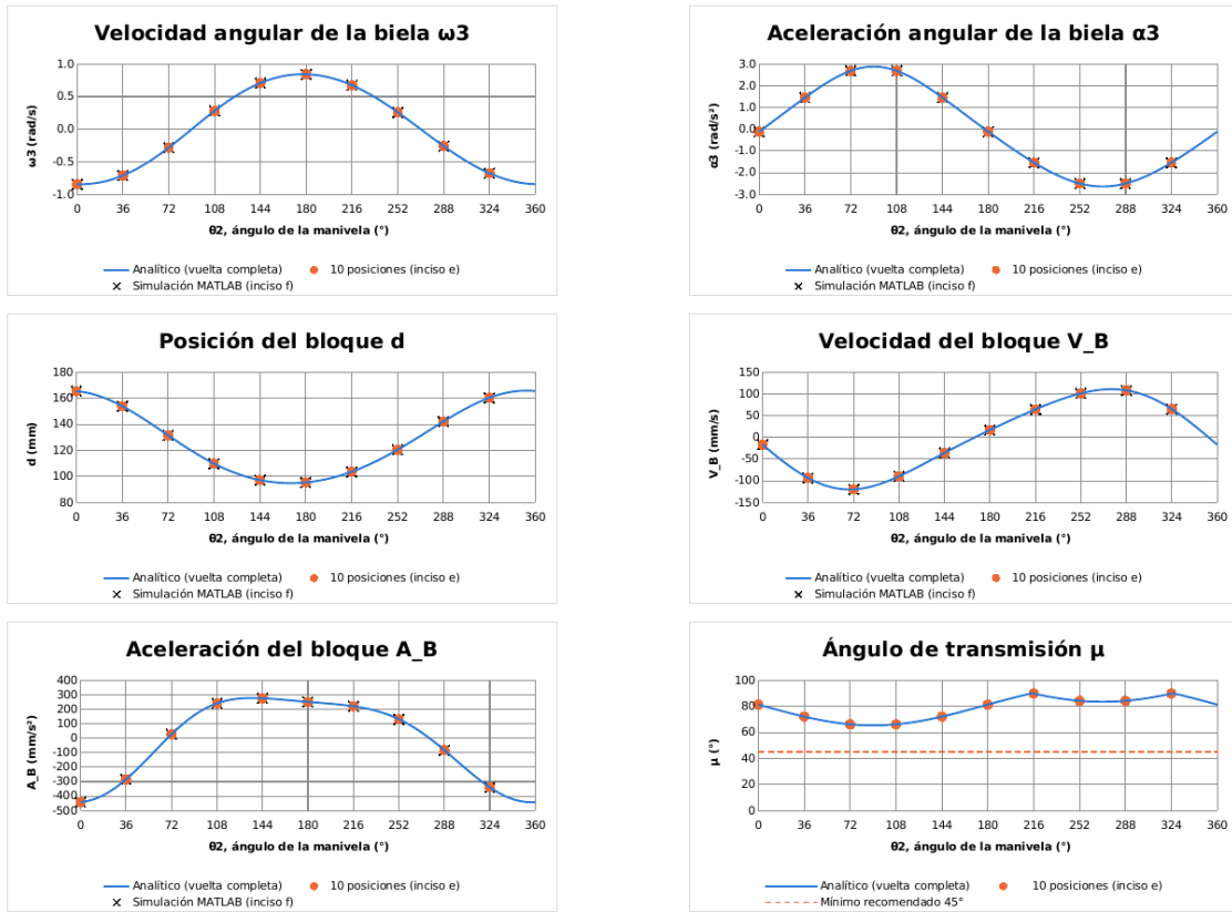
Figura 17. Hoja "P2 Graficas" del Excel: variables del mecanismo en función del ángulo de entrada.
