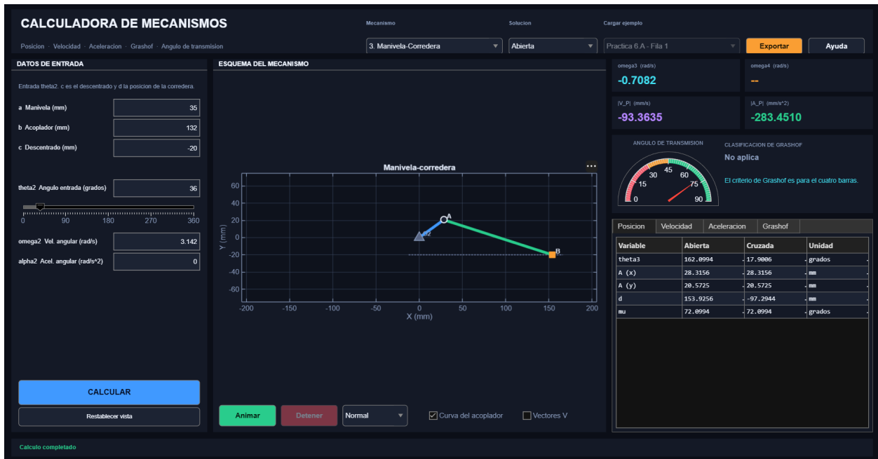
Figura 14. Calculadora de Mecanismos en \theta_2 = 36^\circ (posición 2): mismos valores que el ejemplo resuelto de la posición 2 (Ejemplo resuelto).
